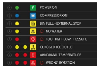
Señalización LED
